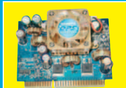
Dual Power System (DPS) – новая технология, обеспечивающая 6-фазную схему питания для большей стабильности.
